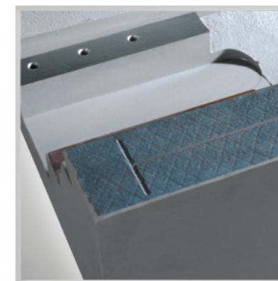
· 贴塑硬轨。
